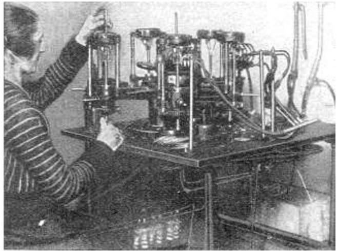
Abb. 4, Einschmelzmaschine
