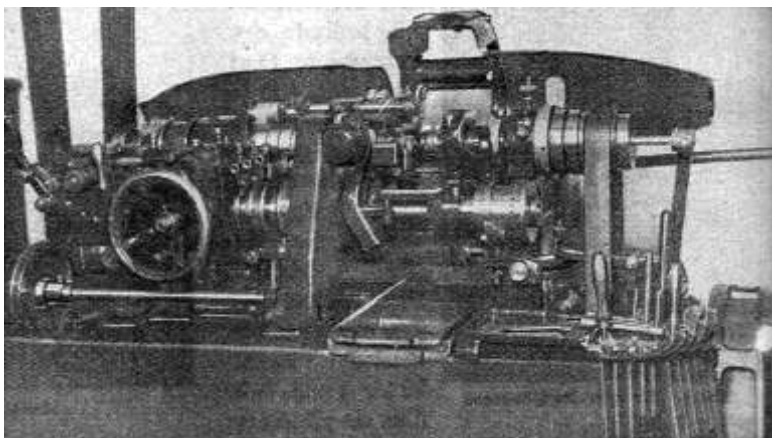
Abb. 8, Bolzenautomat
