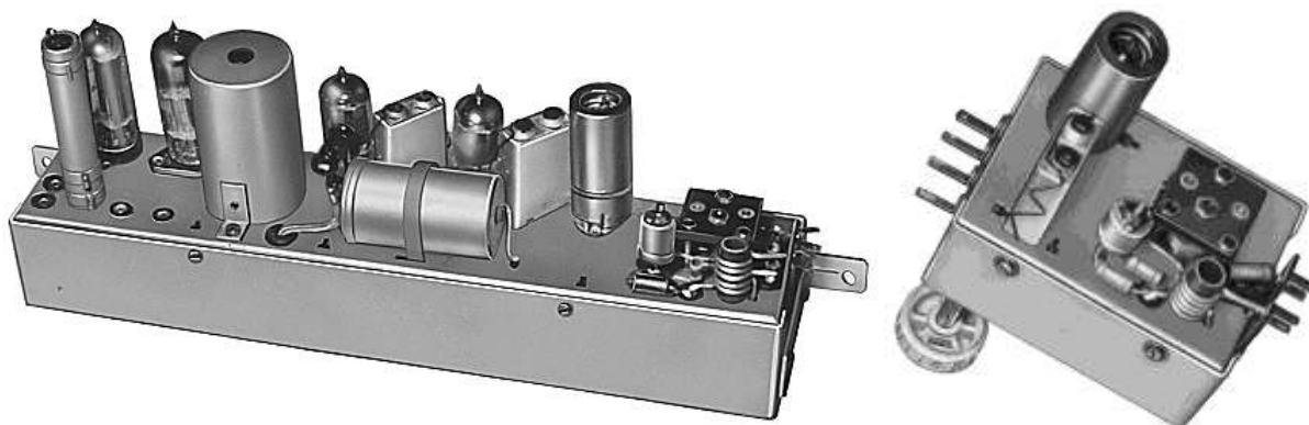
ZEHETNER UKW-Einbauper 554 U (links) und UKW-Superaggregat (rechts)
