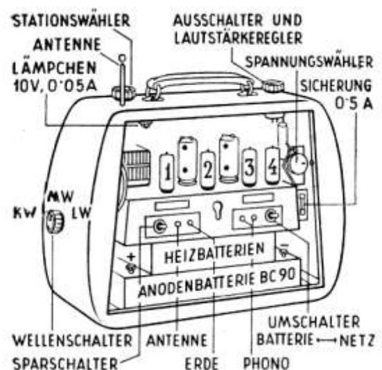
Zeichnung aus der Betriebs- anleitung für den UB 62
