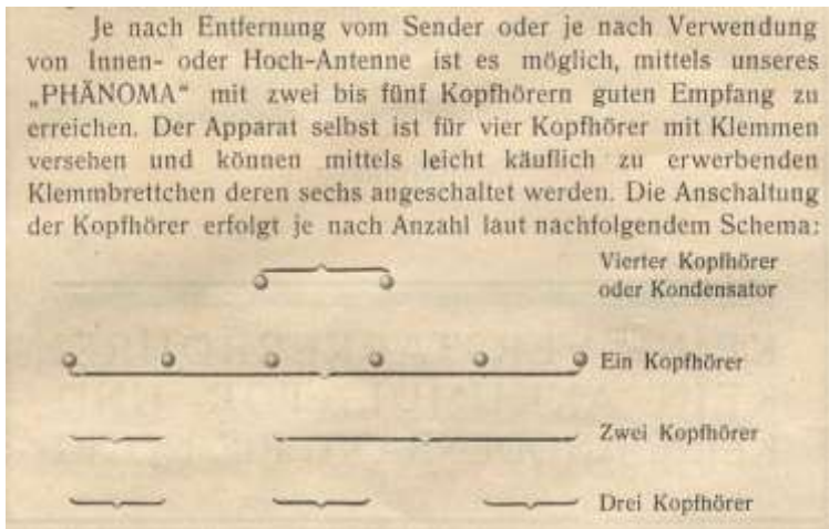
Phänoma - Kopfhörerbeschaltung
