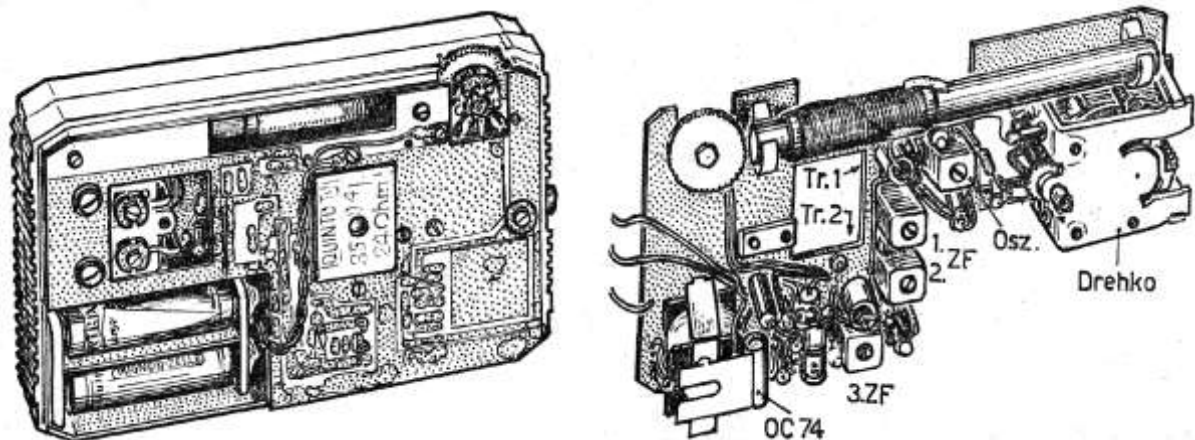
FF-Stern: Zeichnung des Innenaufbaus
