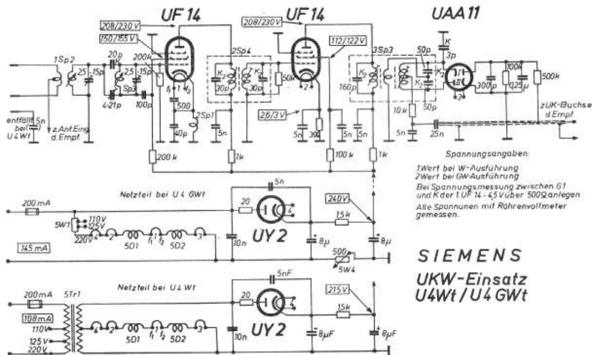
Schaltplan zum Siemens UKW- Einsatz (D)
