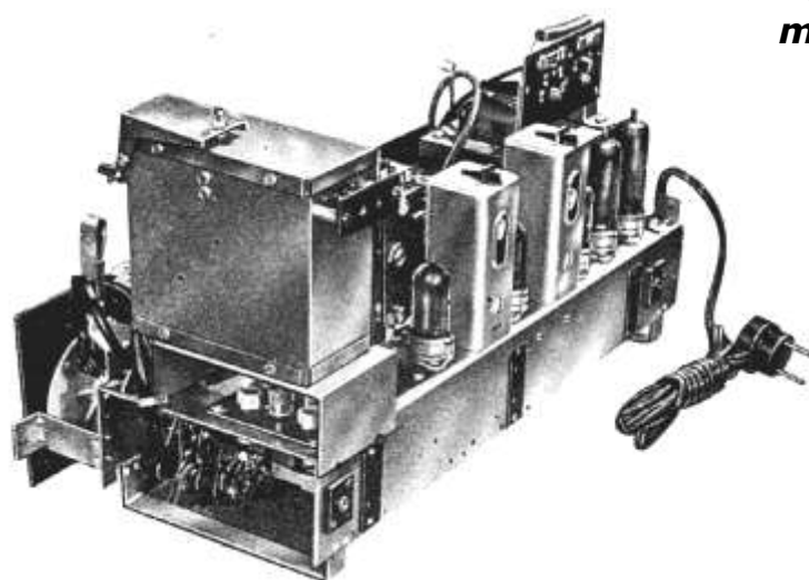
1952: Pendelempfänger Minerva FMP 2, aufgebaut auf dem Chassis des Modells 515 W
