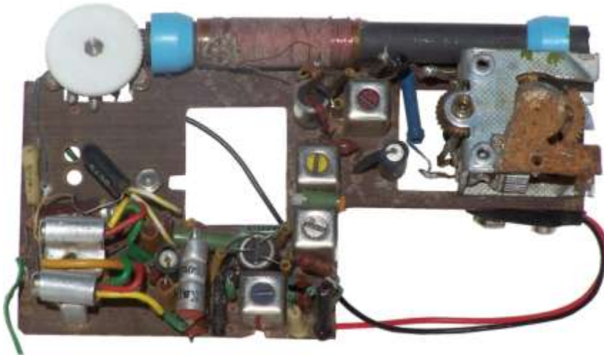
FF-Stern Bauteilseite
