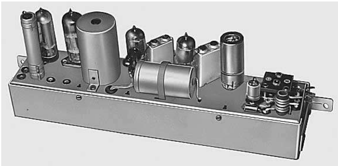
1953: Zehetner „Ultra-UKW-Einbausuper, 454 U oder 554 U“ (4 oder 5 Röhren), Allstrombetrieb. Preis: 680,- bzw. 795,-. Bestückung: EC92, (2x) 12AU6, 19T8, 35W4.
