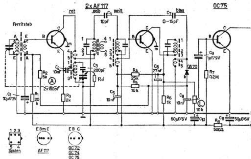
FF-Stern Schaltung: Hochfrequenzteil mit NF.- Vorstufe
