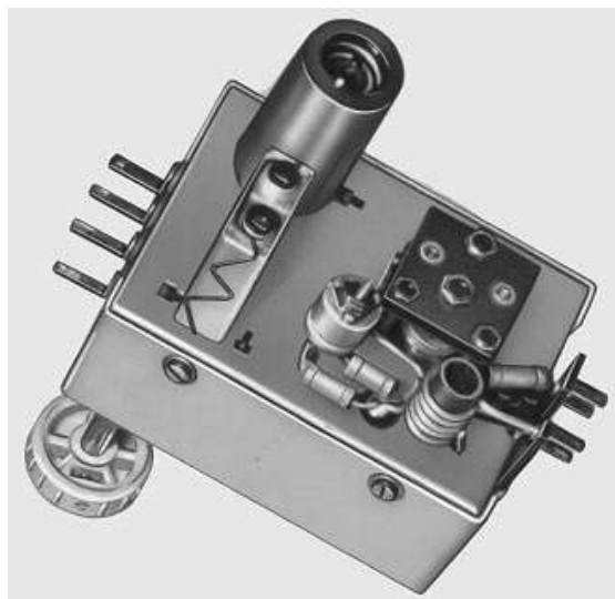
1953: Zehetner „Ultra-UKW-Superaggregat“. UKW-Tuner mit EC 92, Drehkoabstimmung, Preis: 215,-
