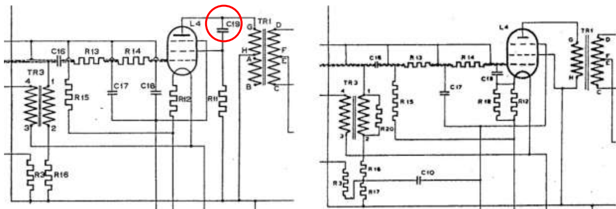
Schaltungsauzug erste NF-Stufe: Phi1UK41 (links),
