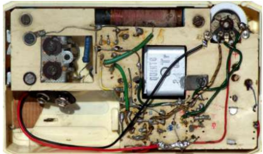
FF-Stern Lötseite
