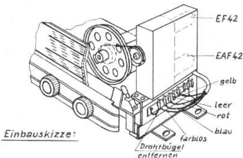
1952: Einbauskizze für den C & N UKW-Pendler
