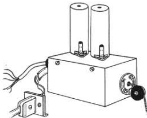
1953: Ansichtszeichnung des Kapsch- Pendlers
