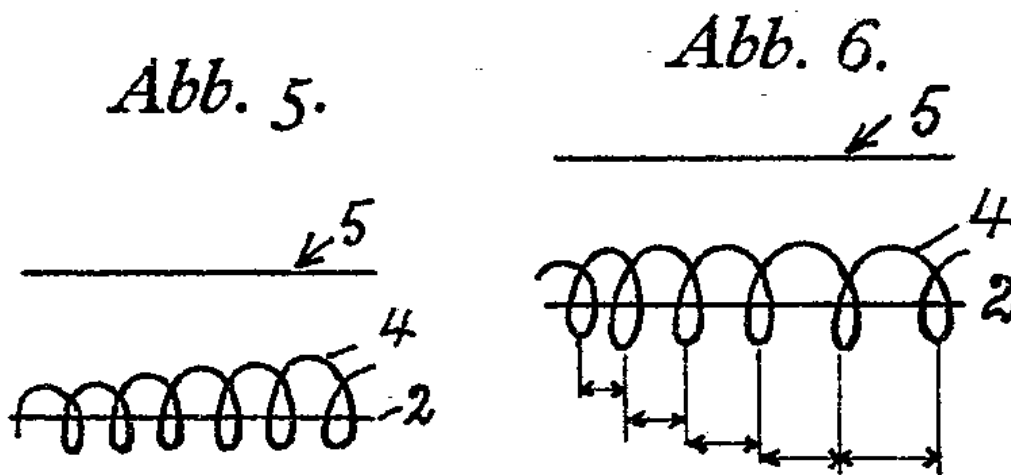
Abb.5 und 6. Aus dem D.R.P. 398.864 von Huth
