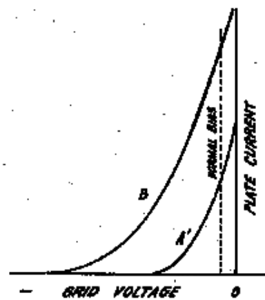
Abbildungen aus U.S. Pat. Nr. 2.066.284 von Ballantine
