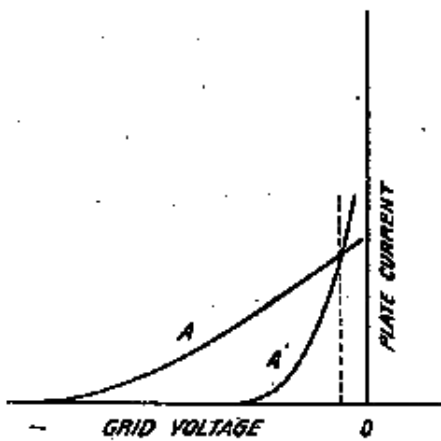
Abbildungen aus U.S. Pat. Nr. 2.066.284 von Ballantine
