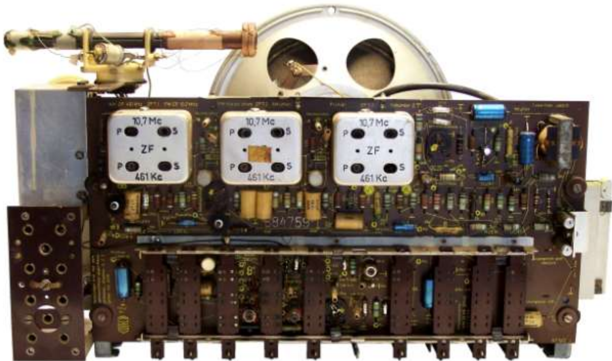
MINERVA Minola Cordless 603, Chassis Rückansicht
