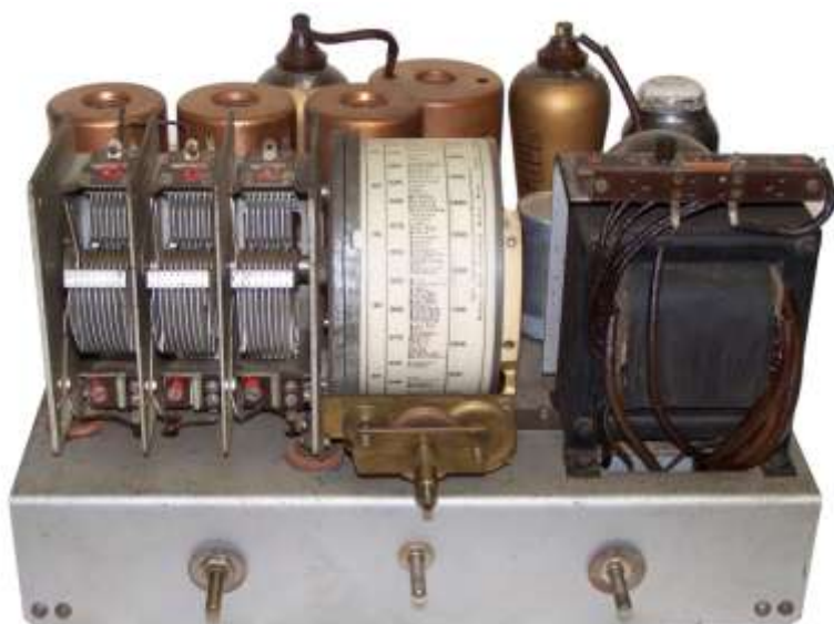
Austro-Super Chassis, Vorderansicht
