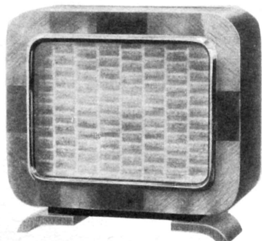
Links: Ein neuer Dynamischer, Blaupunkt 72 D
