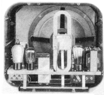
Neufeldt & Kuhnke bleibt beim beliebten Farrand-Inductorlautsprecher und baut ihm ins Gehäuse einen Wechselstromzweier ein.
