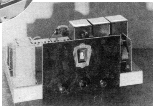
Ein Bandfiltersuperhet, der in Baukastenform erscheint: Schalecohet
