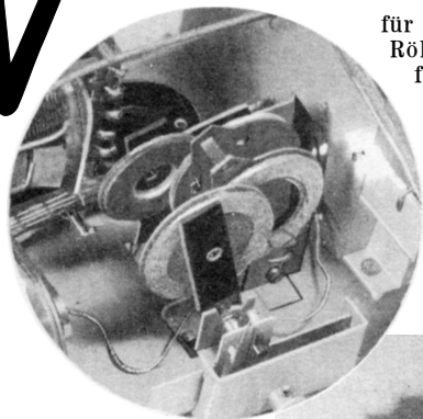
Flachspulen in den neuen Telefunken- geräten.
