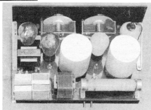
4-Röhren-Schirmgitter-Gleichstromempfänger der Feinmechanik A.G.
