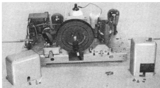
Der Telefunkenvierer bietet erstklassige Werkmannsarbeit.
