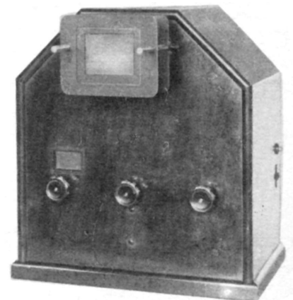
Nipkowscheiben - Projektionsempfänger für 4800 Bildpunkte der Fernseh A. G.
