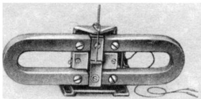
„Tonofox“, ein wegen seiner Einstellmethode sehr interessantes System
