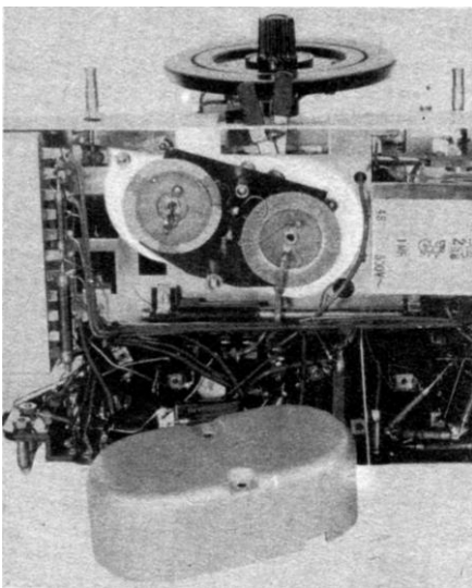
Ein Blick in die geöffnete Boxe, in der die Spulen — für den zweiten Abstimmkreis sitzen. —
