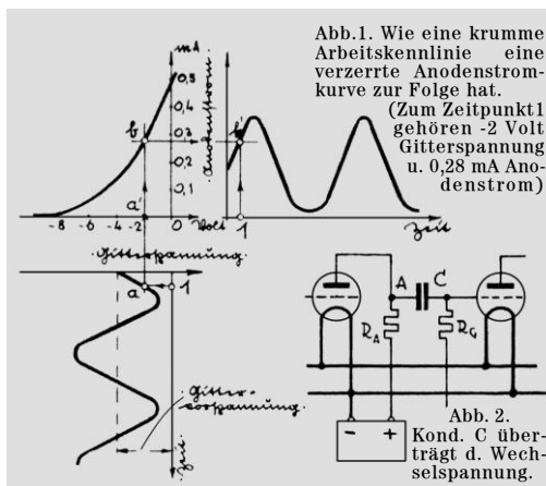
Abb. 1. Wie eine krumme Arbeitskennlinie eine verzerrte Anodenstromkurve zur Folge hat. (Zum Zeitpunkt 1 gehören -2 Volt Gitterspannung u. 0,28 mA Anodenstrom)
