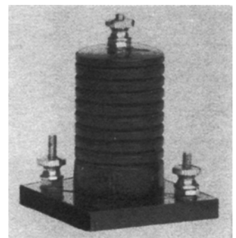
HF-Drossel mit eingebautem 300-cm-Block, eine praktische Neuerung der A. P.W.
