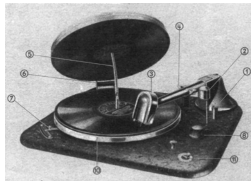
Ein höchst einfacher und zuverlässiger automatischer Plattenwechsler von Körting.
