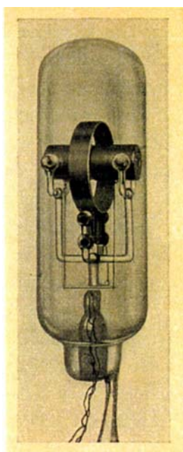
Bild 80. Glimmentladungs-Verstärker nach Kossei mit Kanalstrahlen – Steuerung durch ein Hilfsfeld.
