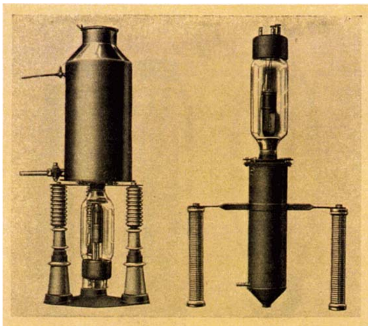
Bild 91. Aus der Entwicklung der wassergekühlten Senderöhren: Links erste Ausführung mit Siedekühlung, Verbindung von Metall und Glas mittels Platinring (1918), rechts fortgeschrittenes Stadium mit Durchflußkühlung, Glas unmittelbar mit Kupferring verschmolzen (1920).
