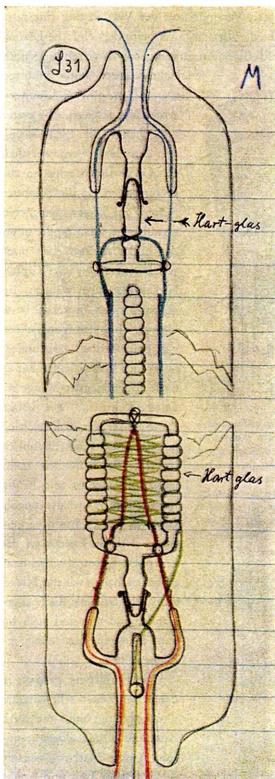
der ersten Zeit der Entwicklung, Wiedergegeben nach einer Handzeichnung von Hans Rukop in einem Typenbuch des Telefunken-Röhrenlaboratoriums (1915 bis 1918).
