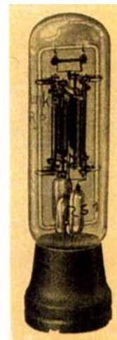
Bild 85. Erste Senderöhre Telefunkens, RS 1, mit etwa 3 Watt Hochfrequenzleistung bei 440 Volt Anodenspannung. Erzeugnis der Fabrik Friedrichstraße. Modell für Schützengrabensender. Man beachte den komplizierten Bau des Elektrodensystems.
