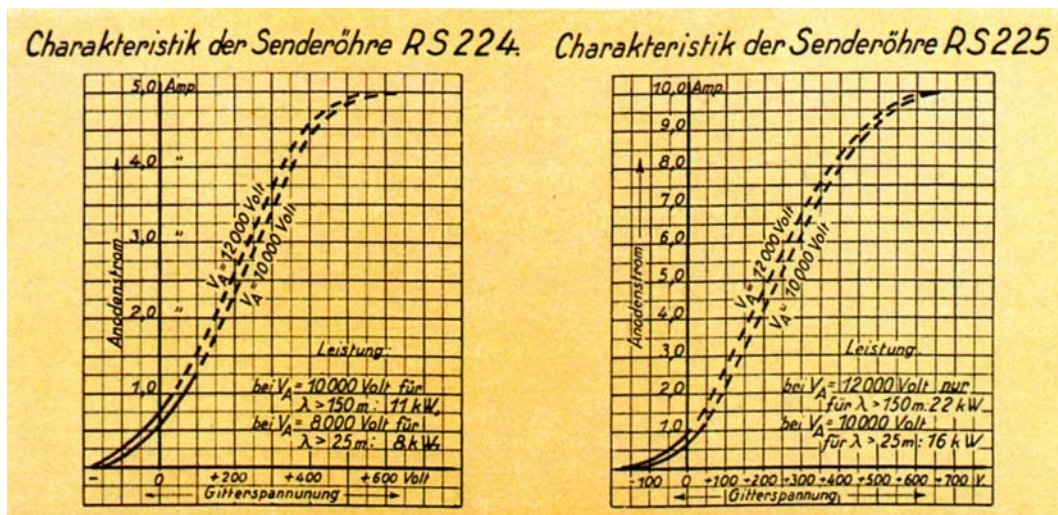
Bild 107. Kennlinien der Wasserkühlsenderöhren RS 224 und RS 225.
