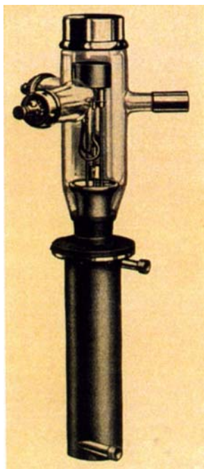
Bild 96. Wassergekühlte Hoch- und Gleichrichterröhre für 10000 Volt, Typ RG 221, für hohe Gleichstromleistungen. Ersetzt je mehrere der bei den großen Sendern bisher gebräuchlichen luftgekühlten Glasventilröhren.
