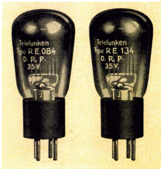
Bild 72. Rundfunkröhrentypen RE 084 und RE 134 mit nach dem Dampfverfahren hergestellter Kathode. Beispiele modernster Hochemissionsröhren, 30 und 50 Milliampere Sättigungsstrom.
