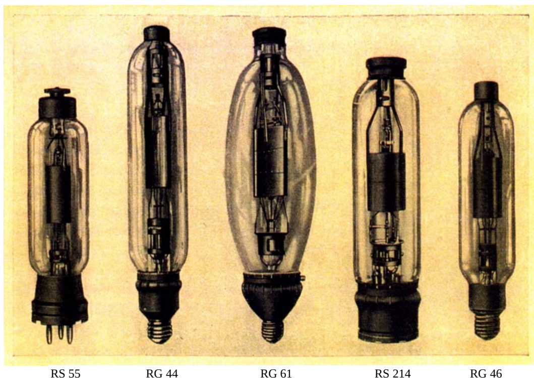
Bild 90. Entwicklungsreihe von luftgekühlten Hochvakuumventilen (neben Senderöhren). Zur Lieferung von hochgespanntem Gleichstrom für Röhrensender.
