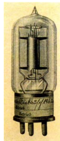
Bild 74. Röhre mit Raumladungsgitter RE26 , Telefunken-Doppelgitterrohr in früherer Ausführung mit Wolframfaden.
