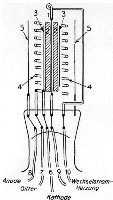
Bild 75. Innenaufbau der indirekt geheizten Rundfunkempfangsröhre Type REN 1104 für Netzanschluß. Die Kathode 3 ist vom wechselstromdurchflossenen Heizdraht 1 mittels des elektrisch, aber nicht thermisch isolierenden Rohres 2 vollkommen getrennt, wodurch ein geräuschloses Arbeiten des Verstärkers erzielt wird.
