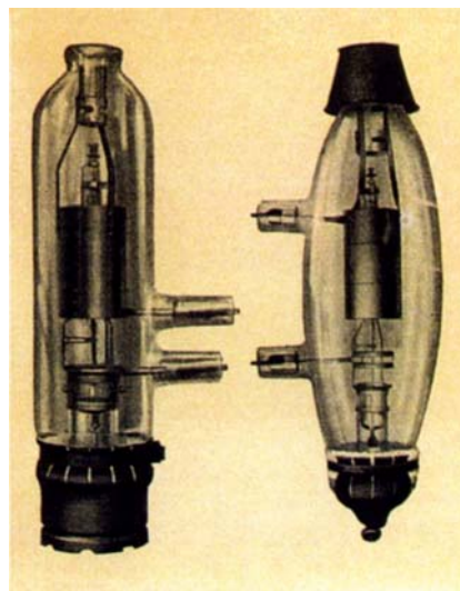
Bild 98. Luftgekühlte Kurzwellensenderöhre RS 207 für etwa 1,5 Kilowatt. Bauweise wie bei RS 229, nebenstehendes Bild. Oben aufgesetzt eine Metallkappe als statischer Schutz gegen dielektrische Beanspruchung des Glases. Leistungs-Vorstufenröhre moderner Kurzwellensender. Maßstab gegenüber Bild 97 stark verkleinert.
