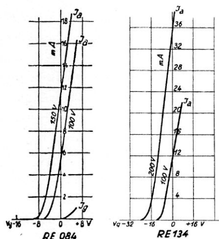
Bild 73. Kennlinien der Rundfunkempfangsröhren RE 084 und RE 134. Große Steilheit, 2 Milliampere/Volt, Durchgriff 6% und 10%.
