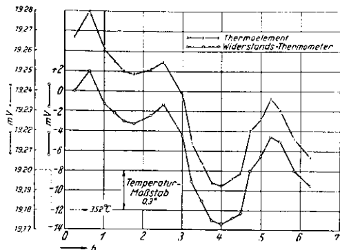
Bild 9. Ergebnis einer Temperaturmessung mit Widerstandsthermometer.
