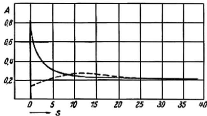
Bild 3. Einschaltvorgang; — ohne Urdox-Widerstand, - - - mit Urdox-Widerstand.
