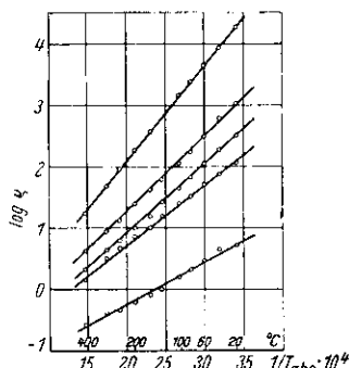
Bild 1. Widerstands-Temperatur-Kurven, gemessen an Mg-Ti-Spinellkörpern.
