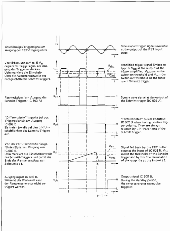
Abb. 12: Signalablauf im Zeitablenkgenerator (getriggelter Betrieb)
