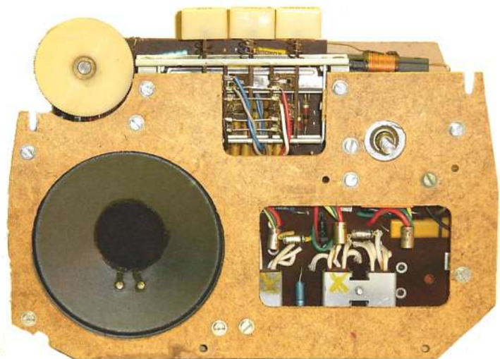
Chassisansicht von vorne
