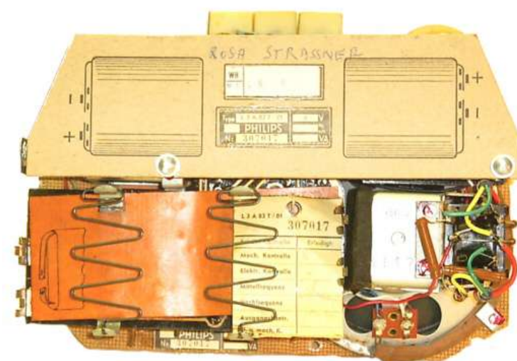
Chassisansicht von hinten
