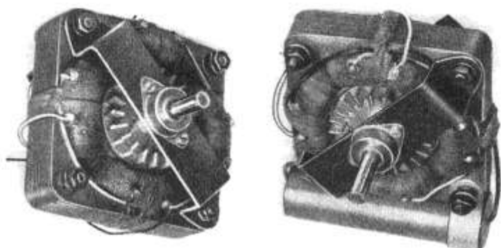
Ansicht der beiden Laufwerksmotoren
