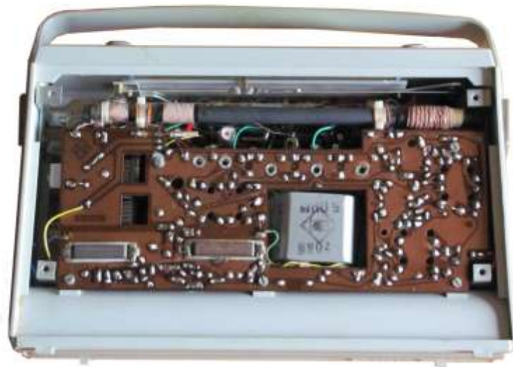
Rückansicht mit Blick auf die Lötseite der Printplatte
