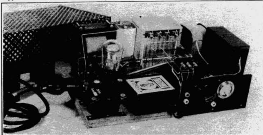
Das fertige Gerät.
