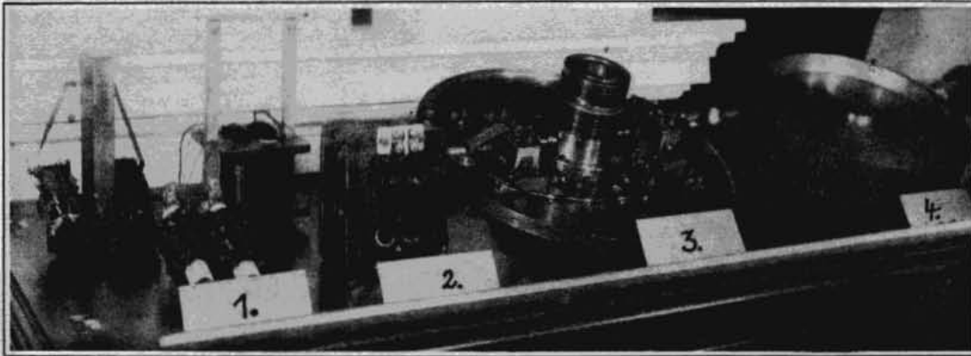
Apparate für einen Hochfrequenzmaschinensender. — Phot. Saulmann & Wessel
