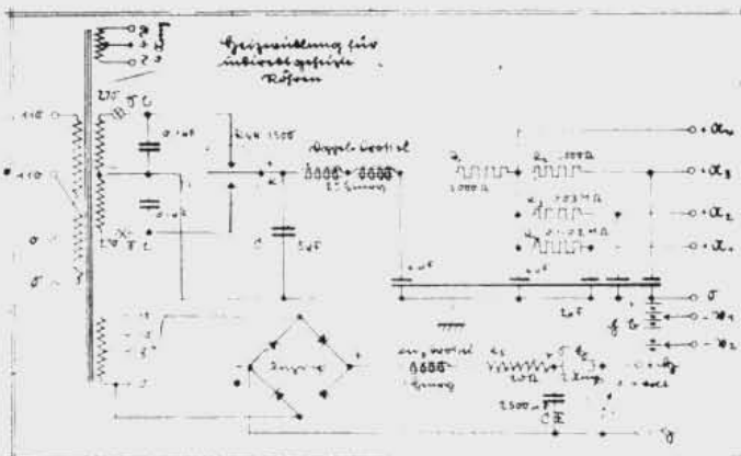
Die Prinzipschaltung unserer Wechselstrom-Heizanode
