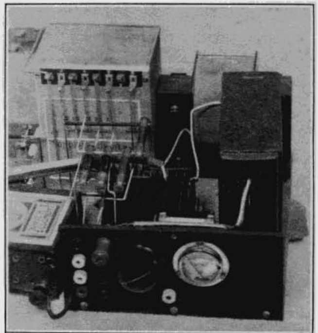
Vorne das Anschlußbrettchen, dahinter das Kuproxsystem, daneben der Trockenelektrolytkondensator, ganz hinten die Netzdrossel und der Kondensatorenblock.
