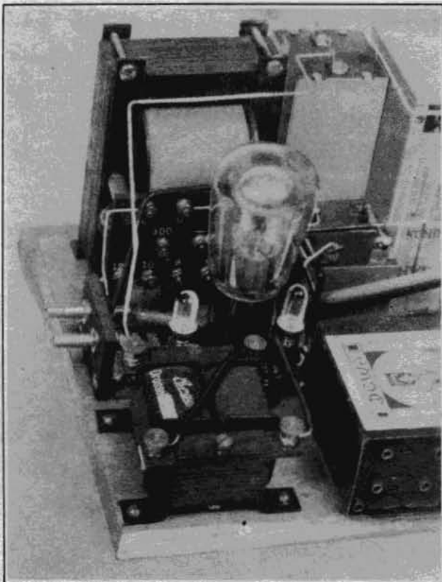
Der Gleichrichterteil. Im Hintergrund der Netztrafo, in der Mitte die Glimmgleichrichterröhre, rechts vorne die Gitterbatterie.
