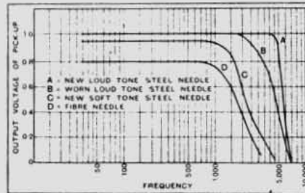
Abb. 9. Das Verhalten eines Pick-ups bei Verwendung verschiedener Nadeln.
