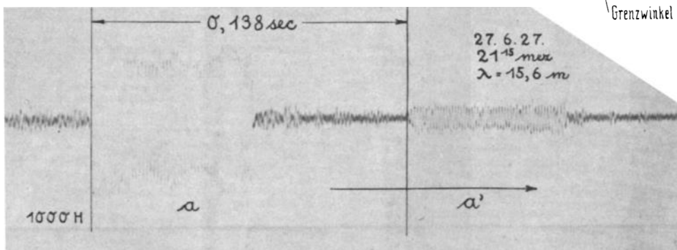
Abb. 2. Mittels besonderer Instrumente (Oszillographen) kann man die elektrischen Wellen sich aufzeichnen lassen und so feststellen, wie oft und in welcher Zeit sie um die Erde gelaufen sind.
