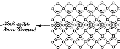
Abb. 6. Wenn sich die Elektrizitätsteilchen im Gänsemarsch vorwärts bewegen, so ist das unser Strom. Die Wirbelteile des Äthers müssen sich dann drehen.
