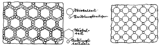
Abb. 1 und 2. Ein Bild von einem Stückchen des Äthers in ungeheurerer Vergrößerung; links genau, rechts etwas vereinfacht.
