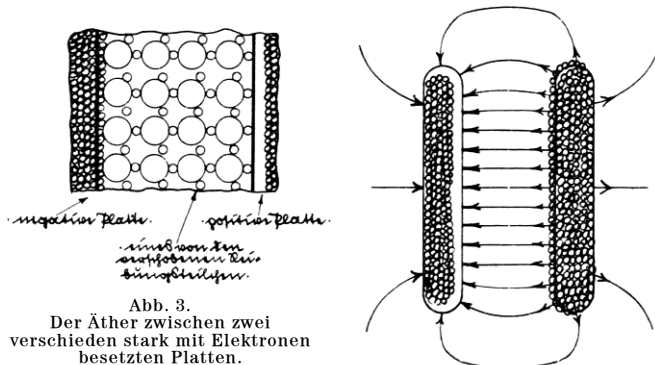
Abb. 4. Die Richtungen der Verschiebung im Äther. Durch die Dichte der Feldlinien ist angedeutet, wo die Verschiebung zwischen den beiden Platten am stärksten ist.
