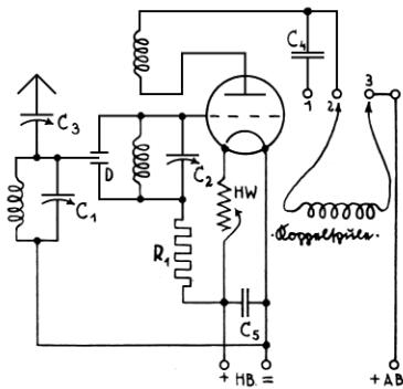
L i n k s : Das Schaltbild des (Tropa-) Vorsatzes.
