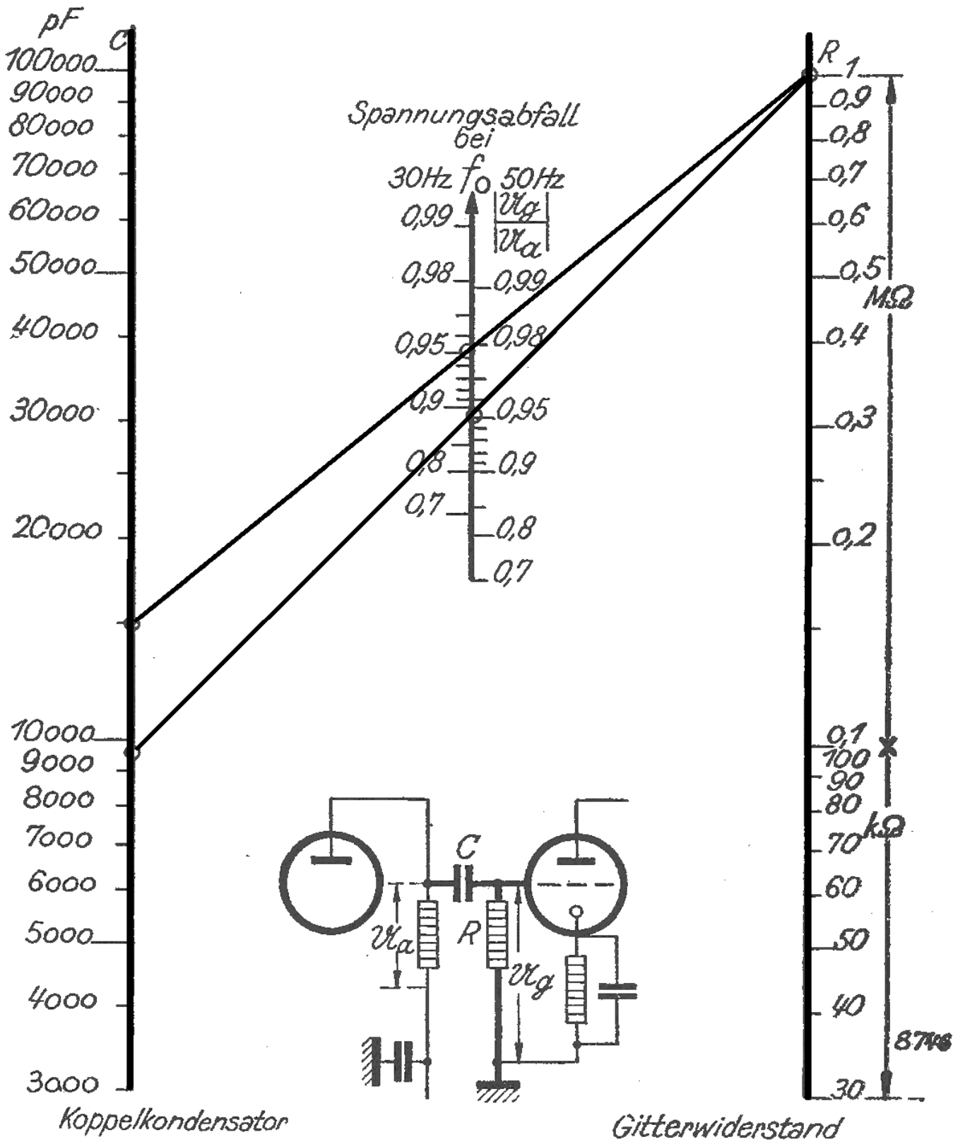
Tafel zur Bestimmung des Koppelkondensators bei Tonfrequenzverstärkern
