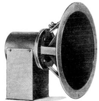
Elektrodynamisches Lautsprechersystem „Hegra“, Fa. Hermann Grau
