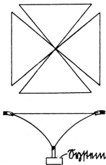
Das Sektorphon von Graß & Worff.
