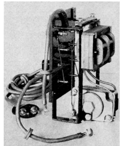
Abb. 5 Die Inneneinrichtung des „Protax“, unten der Trockengleichrichter, darüber die Drossel
