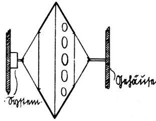
Kompressor des „Eloden“-Lautsprechers
